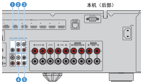
本机（后部）
