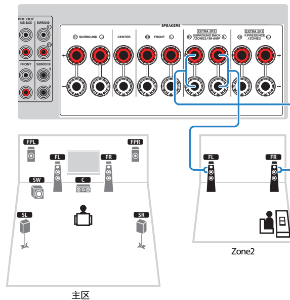
本机（后部）
