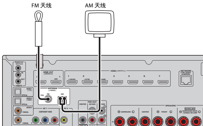
本机（后部）
