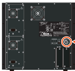
DSP-R10,DSP-RX(-EX) (задняя панель)
