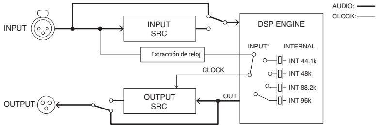
Diagrama de bloques del SRC
